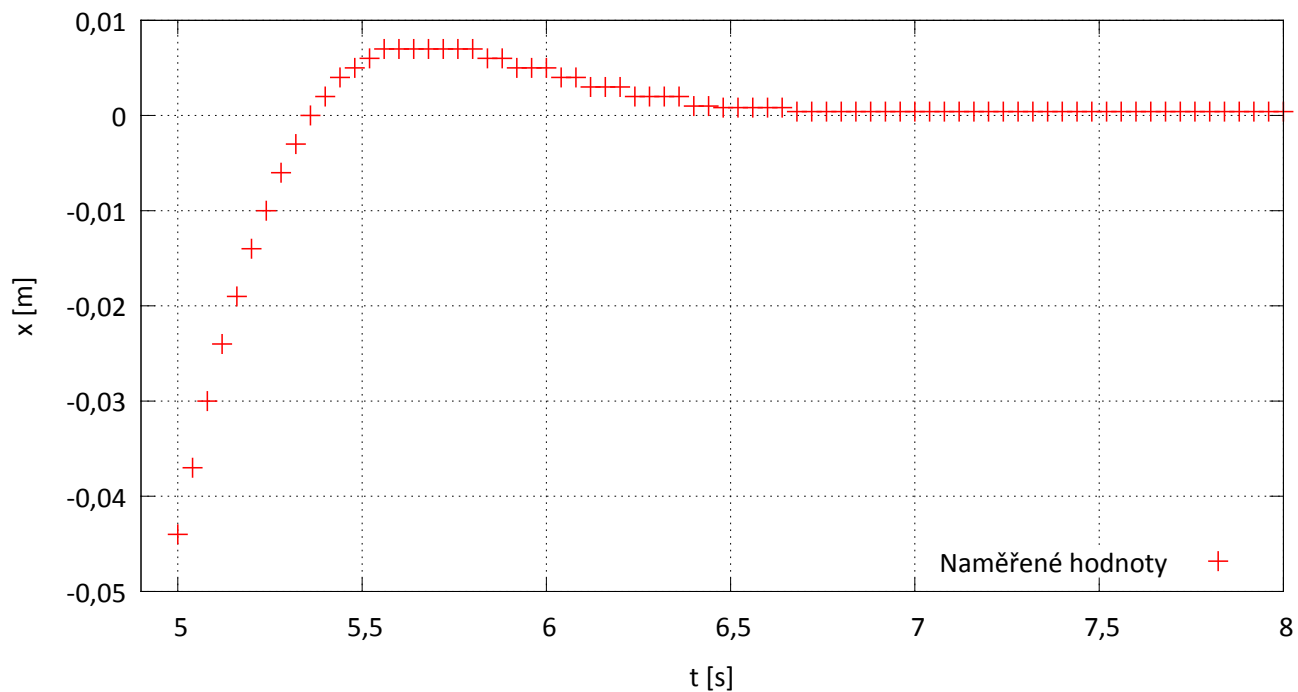
Obr. 9: Graf časového průběhu tlumených kmitů Pohlova kyvadla pro závaží o hmotnosti m = 10 g a tlumícího proudu I = 1,5 A; x je poloha v závislosti na čase t .
