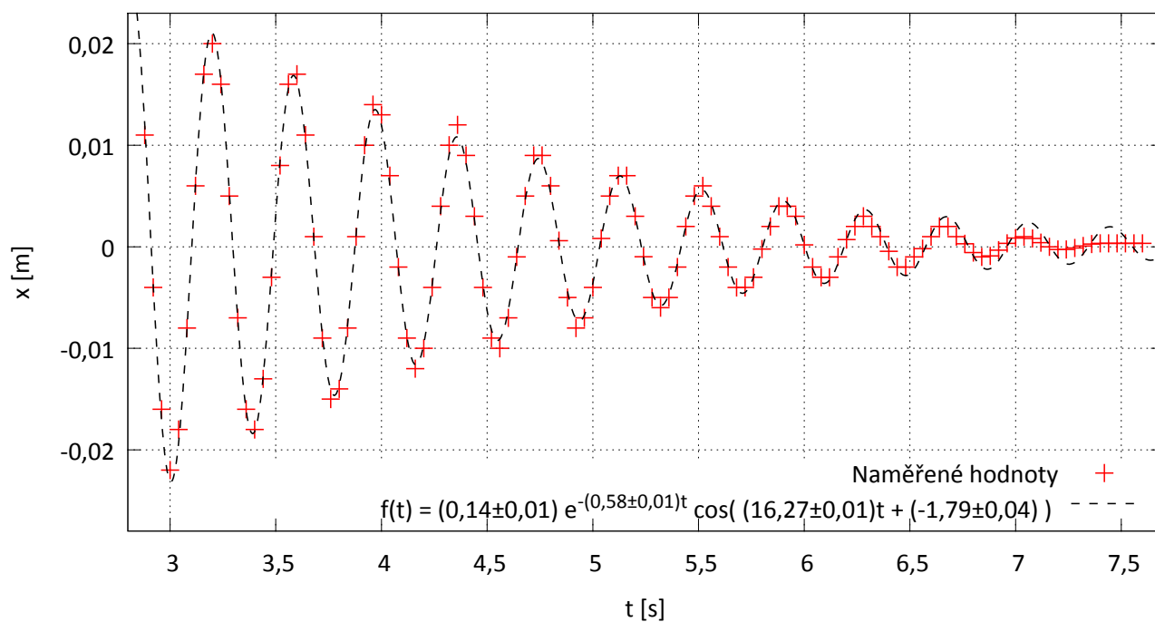
Obr. 1: Graf časového průběhu tlumených kmitů LHO pro závaží o hmotnosti m = 20 g; x je poloha v závislosti na čase t . Naměřené hodnoty jsme proložili podle rovnice (8).
