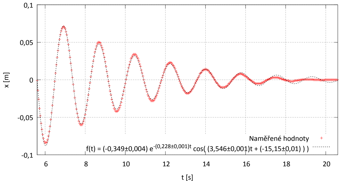
Obr. 6: Graf časového průběhu tlumených kmitů Pohlova kyvadla pro závaží o hmotnosti m = 10 g a tlumícího proudu I = 0,4 A; x je poloha v závislosti na čase t . Naměřené hodnoty jsme proložili podle rovnice (8).
